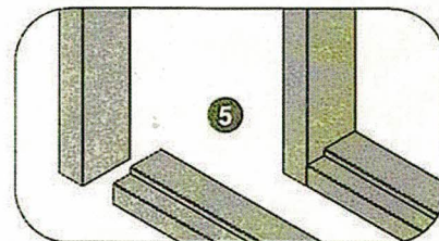
แสดงลักษณะการเชื่อมต่อชน
